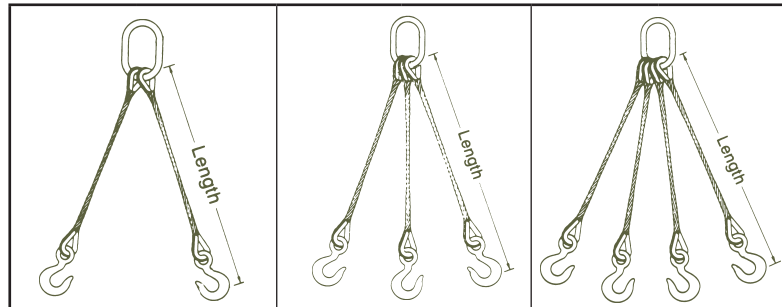
2-Leg Bridle
